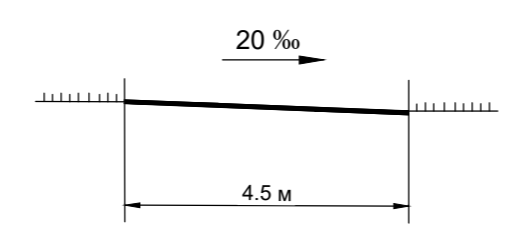
Поперечний профіль проїзду Розріз 1-1
