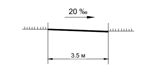
Поперечний профіль проїзду Розріз 2-2
